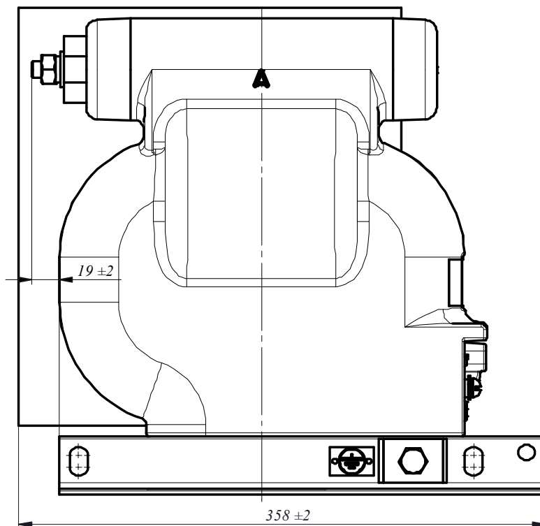
Рисунок А.2 Общий вид трехфазной группы 3x3ZHOЛПМИ (остальное см. рисунок А.1)
